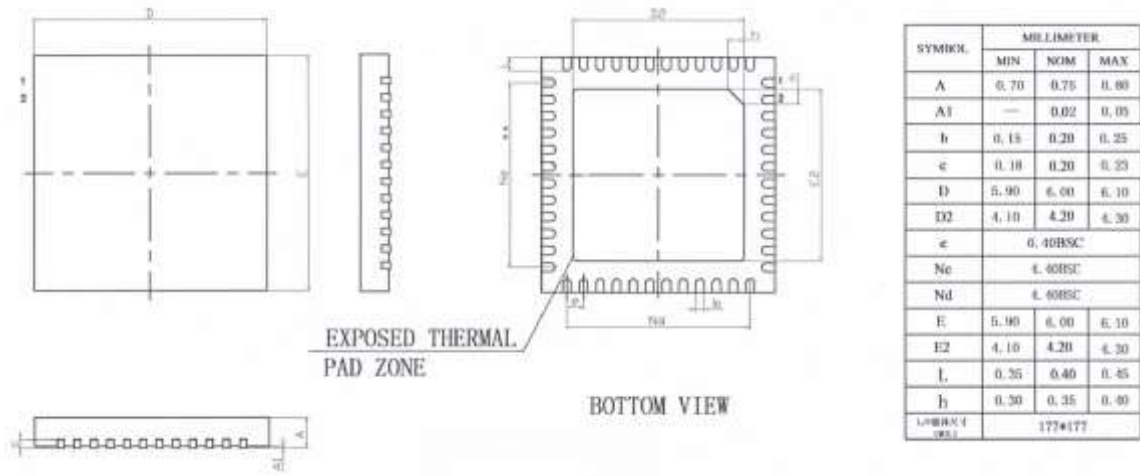
图 1-3 QFN48 外形图
