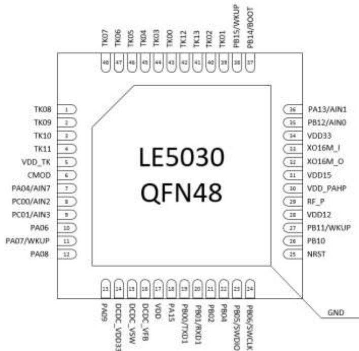
图 1-2 QFN48
